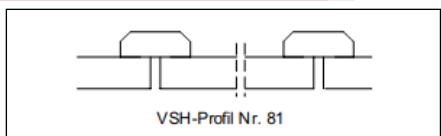
Deckleistenschalung
