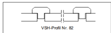
T-Leistenschalung
